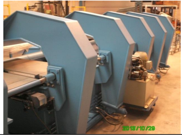
JORNS ML200-SW-RH-SM3-CNC500-6,4 Abkantmaschine von hinten gesehen
